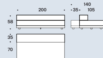
Divano-letto / Sofa-bed
