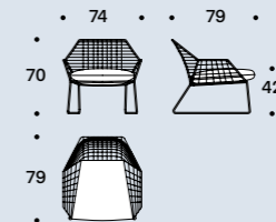
Poltrona / Armchair
