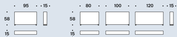
Bracciolo / Armrest - 15
