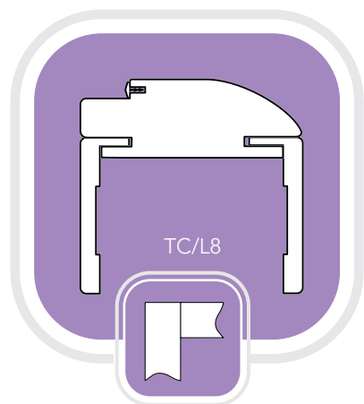
Telaio tondo con coprifili lisci (disponibile solo per porte a vetro)
