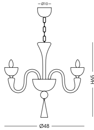
574.3L Lampadario / Chandelier Ø48 cm - H65 cm - catena/chain 50 cm 3 E14 x max 40W 220-240V CE IP20 (1m)
