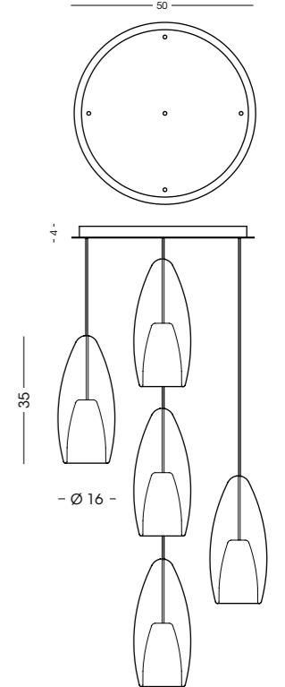
GIG1399.50.5L Plafoniera / Ceiling lamp vetro/glass Ø16 cm - cavo/cable 150 cm 5 E27 x max 105W 220-240V CE IP20 (1m)
