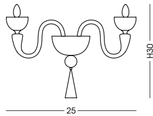
AP571.2L Applique / Wall lamp L25 cm - P25 cm - H30 cm 2 E14 x max 40W 220-240V CE IP20 (1m)
