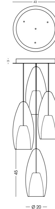
XXL1399.43.4L Plafoniera / Ceiling lamp vetro/glass Ø20 cm - cavo/cable 150 cm 4 E27 x max 105W 220-240V CE IP20 (1m)
