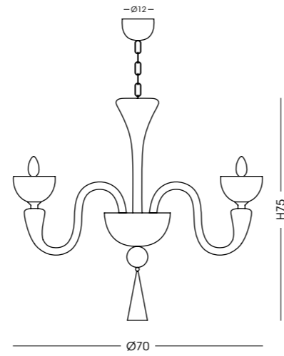
574M.8L Lampadario / Chandelier Ø70 cm - H75 cm - catena/chain 50 cm 8 E14 x max 40W 220-240V CE IP20 (1m)
