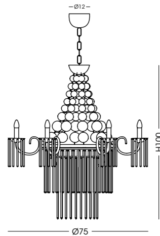
1274.6+4/10L Lampadario / Chandelier Ø75 cm - H100 cm - catena/chain 50 cm 6 E14 x max 40W 4 G9 x max 42W 230V CE IP20 1m
