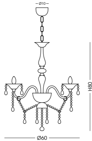
684.3L Lampadario / Chandelier Ø60 cm - H80 cm - catena/chain 50 cm 3 E14 x max 40W 220-240V CE IP20 (1m)
