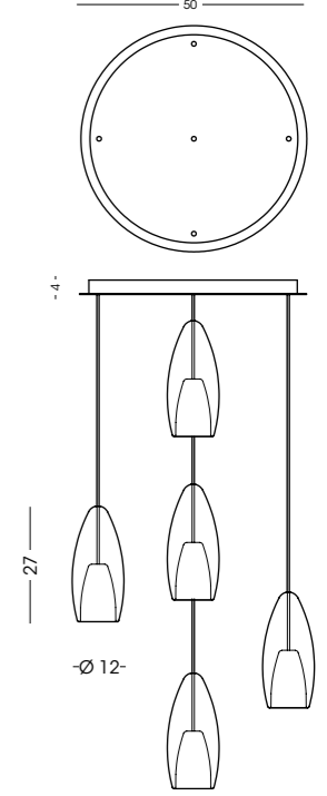
1399.50.5L Plafoniera / Ceiling lamp vetro/glass Ø12 cm - cavo/cable 150 cm 5 E14 x max 60W 220-240V CE IP20 (1m)
