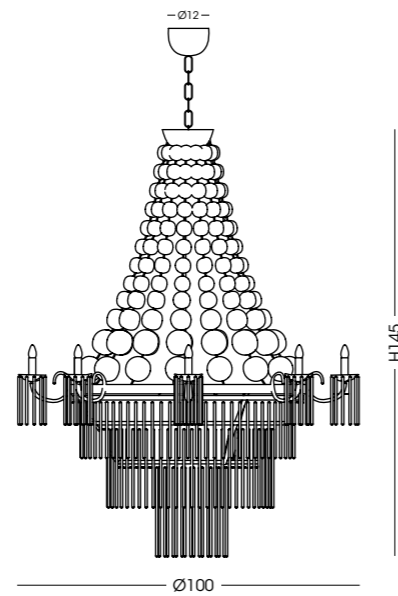
1274.8+8/16L Lampadario / Chandelier Ø100 cm - H145 cm - catena/chain 50 cm 8 E14 x max 40W 8 G9 x max 42W 230V CE IP20 1m
