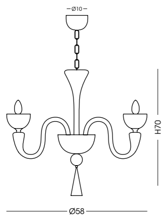
574.6L Lampadario / Chandelier Ø58 cm - H70 cm - catena/chain 50 cm 6 E14 x max 40W 220-240V CE IP20 (1m)
