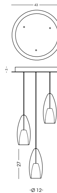
1399.43.3L Plafoniera / Ceiling lamp vetro/glass Ø12 cm - cavo/cable 150 cm 3 E14 x max 60W 220-240V CE IP20 (1m)
