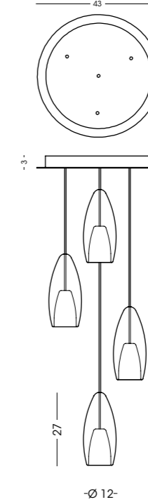
1399.43.4L Plafoniera / Ceiling lamp vetro/glass Ø12 cm - cavo/cable 150 cm 4 E14 x max 60W 220-240V CE IP20 (1m)
