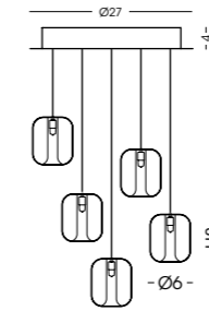
744.5L Plafoniera / Ceiling lamp vetro/glass Ø6 cm - cavo/cable 150 cm 5 G9 x max 42W 230V CE IP20 1m
