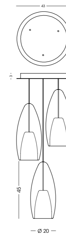
XXL1399.43.3L Plafoniera / Ceiling lamp vetro/glass Ø20 cm - cavo/cable 150 cm 3 E27 x max 105W 220-240V CE IP20 (1m)
