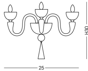
AP571.3L Applique / Wall lamp L25 cm - P30 cm - H30 cm 3 E14 x max 40W 220-240V CE IP20 (1m)
