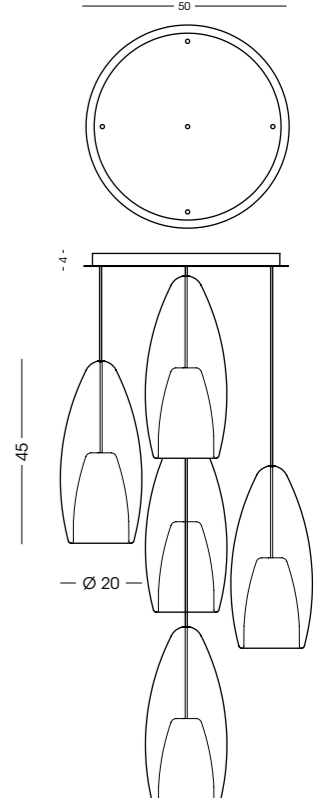
XXL1399.50.5L Plafoniera / Ceiling lamp vetro/glass Ø20 cm - cavo/cable 150 cm 5 E27 x max 105W 220-240V CE IP20 (1m)
