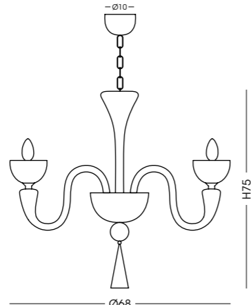
574M.6L Lampadario / Chandelier Ø68 cm - H75 cm - catena/chain 50 cm 6 E14 x max 40W 220-240V CE IP20 (1m)
