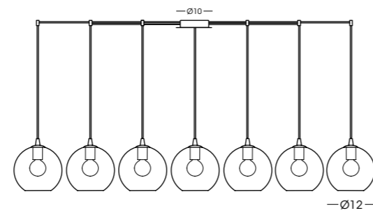
933.7L Sospensione / Hanging lamp vetro/glass Ø12 cm - cavo/cable 250 cm
