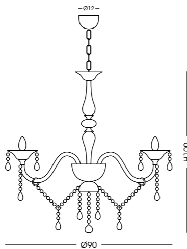
684.8L Lampadario / Chandelier Ø90 cm - H100 cm - catena/chain 50 cm 8 E14 x max 40W 220-240V CE IP20 (1m)
