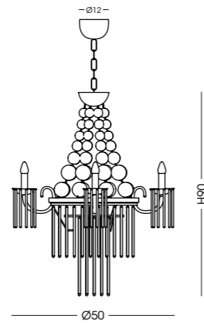
1274.3+4/7L Lampadario / Chandelier Ø50 cm - H90 cm - catena/chain 50 cm 3 E14 x max 40W 4 G9 x max 42W 230V CE IP20 1m
