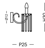
AP1271.1L Applique / Wall lamp L15 cm - P25 cm - H30 cm 1 E14 x max 40W 220-240V CE IP20 1m
