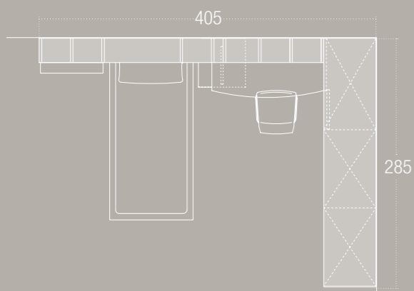
PROPOSTA COMPOSIZIONE T117 L. 405 P. 285 H. 255 cm.
