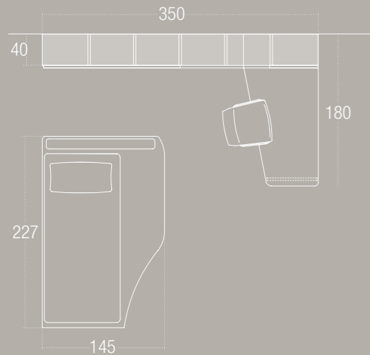
PROPOSTA COMPOSIZIONE T118 L. 350 P. 296,4 H. 220 cm.
