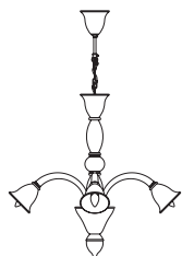
Laguna lampadario 4L BB Ø 73 cm - H 68 cm 4 x E14 40W
