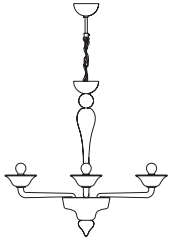
Ca' d'Oro lampadario 3L Ø 81 cm - H 68 cm 3 x E14 40W
