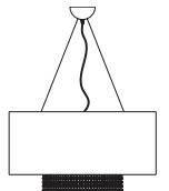
Crystal Shade Ø 70 Ø 70 cm - H 38 cm 3 x E27 40W
