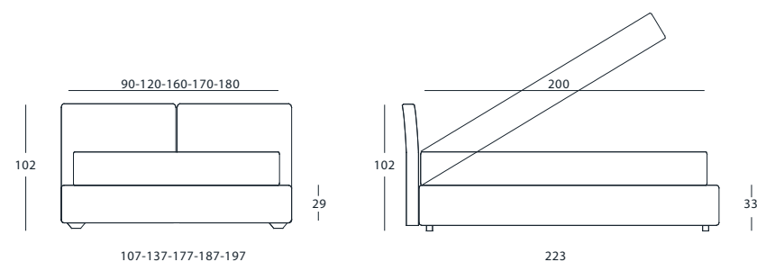
VERSIONE BOX
