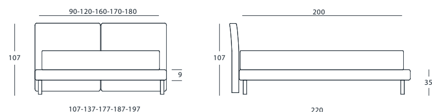
VERSIONE H 9
