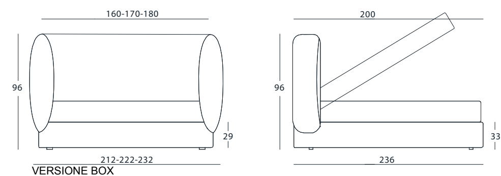
VERSIONE BOX
