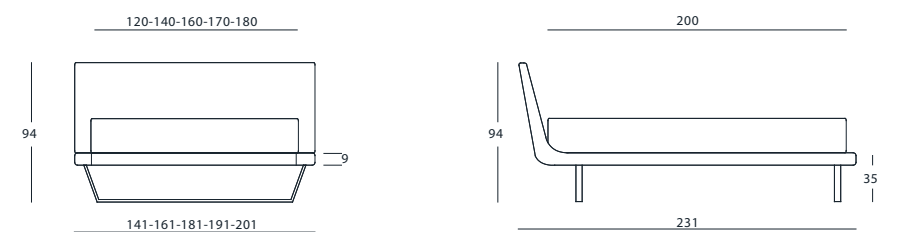
VERSIONE SLITTA
