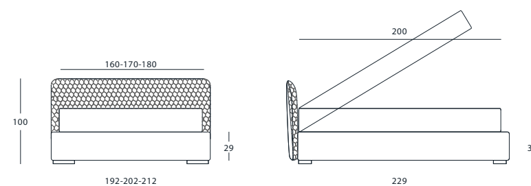
VERSIONE BOX
