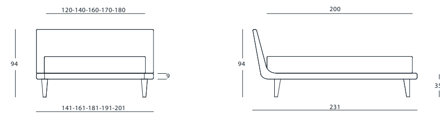
VERSIONE PIEDINI
