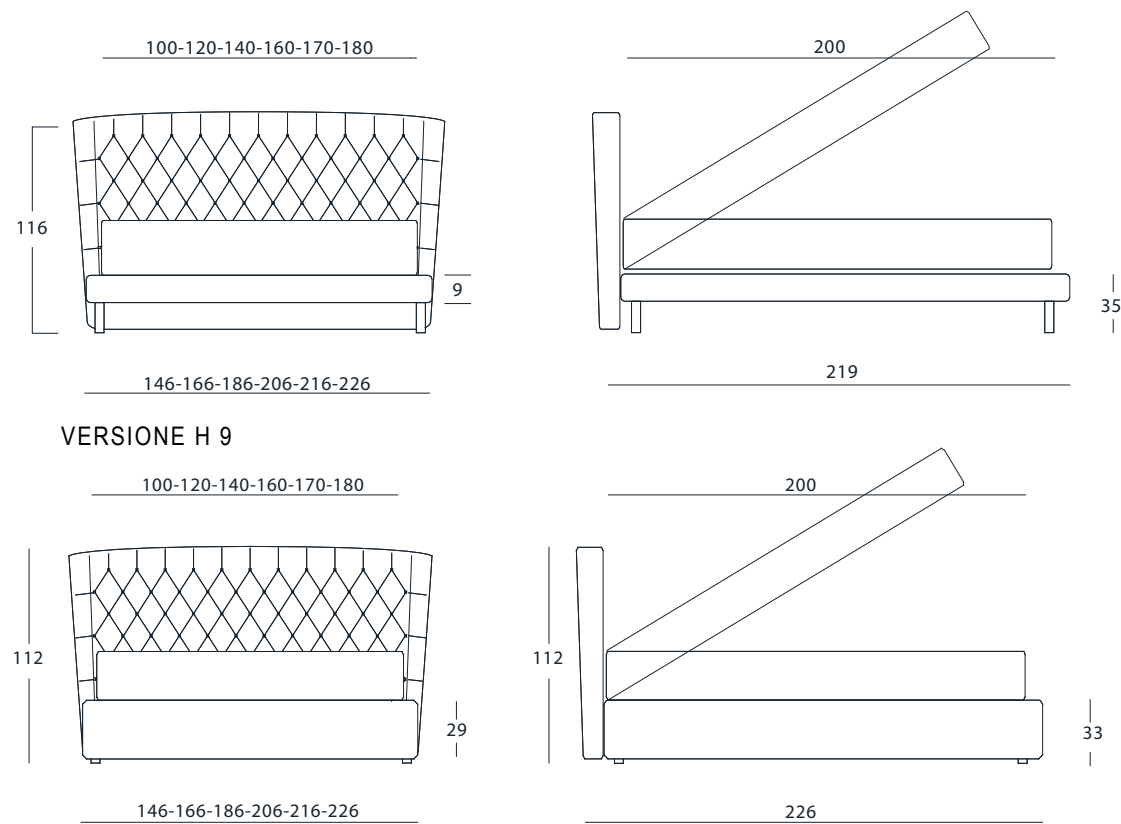
VERSIONE BOX
