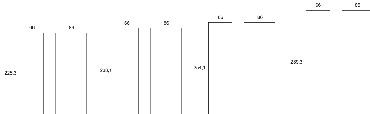
SCHIENALI P. 1,8 cm BACK PANELS D. 1,8 cm
