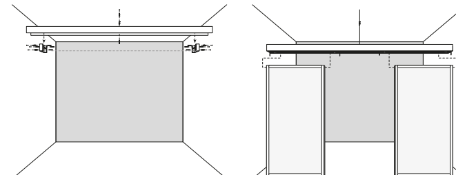
FISSAGGIO BINARIO A 2 VIE SOSPESO PER LARGHEZZA SUPERIORE A 300 CM 2-WAY SUSPENDED RAIL FIXING FOR WIDTH ABOVE 300 CM
