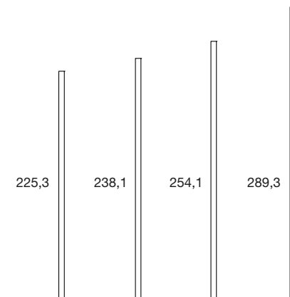
CORNICI TERMINALI P. 5,5 cm END FRAMES D. 5.5 CM
