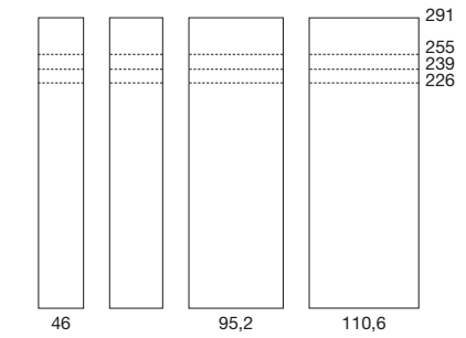
DIMENSIONE MODULI UNIT DIMENSIONS
