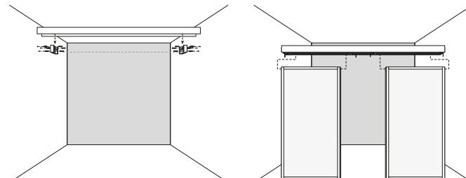
FISSAGGIO BINARIO A 2 VIE SOSPESO PER LARGHEZZA FINO A 300 CM 2-WAY SUSPENDED RAIL FIXING FOR WIDTH OF UP TO 300 CM
