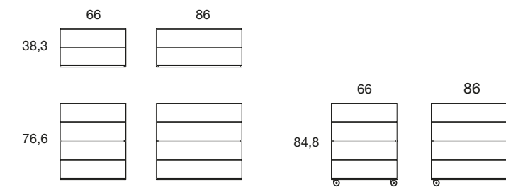
CASSETTIERE P. 48,5 cm DRAWER UNITS D. 48,5 cm
