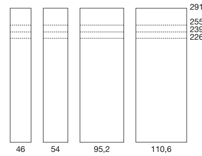
DIMENSIONE MODULI UNIT DIMENSIONS
